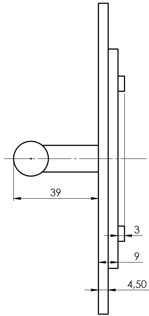
Excel okenní rozvora
